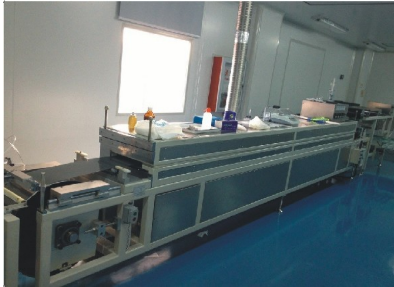
钢带流延机
